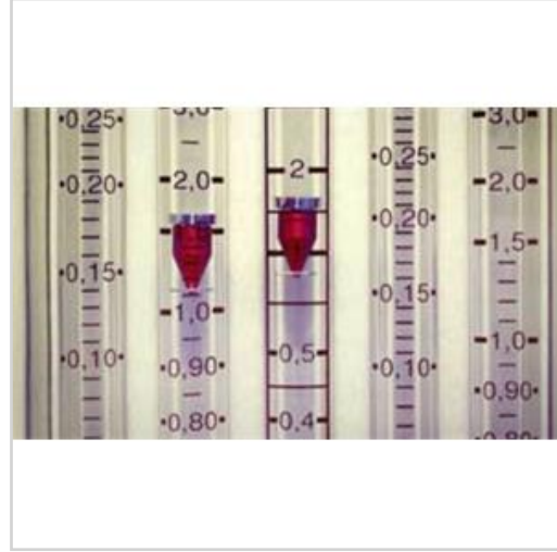
Debimetre Kalibrasyonu
