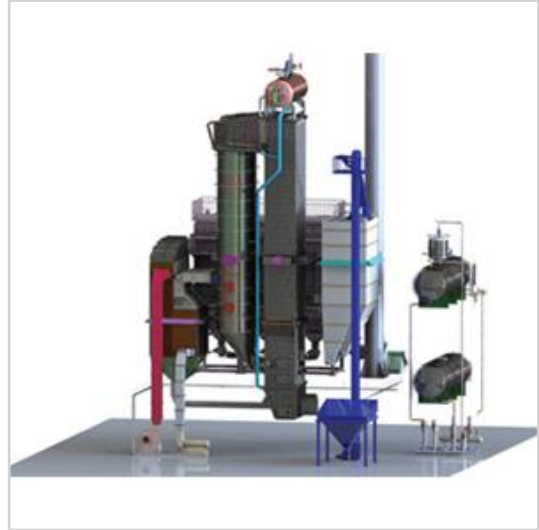
Dolaşım Tip Akışkan Yataklı Buhar Kazanı
