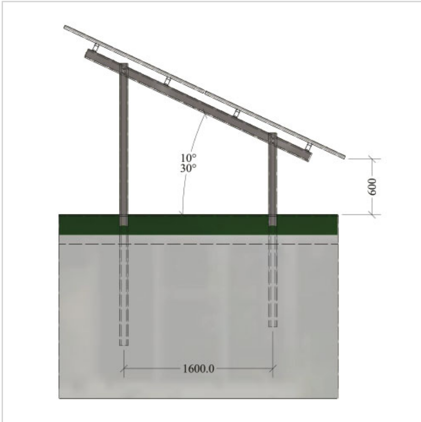
Arazi Tipi Solar Montaj Sistemleri
