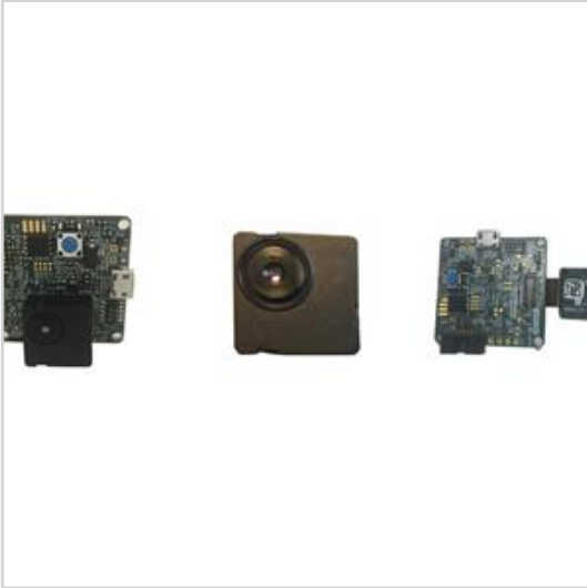
Kamera Çekirdeği İçin Değerlendirme Kiti (EV-MSCC0835 - LWIR)
